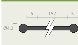
RP381 solid EPDM
